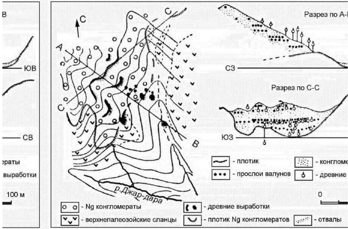
Рис. 6. План и разрезы древних разработок неогеновых конгломератов (р. Джар-дара) (по В.И.Попову)
