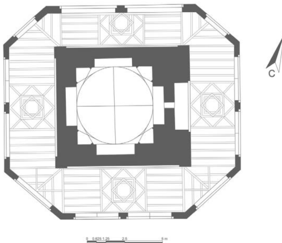
Расми 36. Тарҳи меъмории мақбараи Мавлоно Тоҷиддин (акс аз бойгонии шуъбаи бостоншиносии Институти таърих, бостоншиносии ва мардумшиносӣ )
