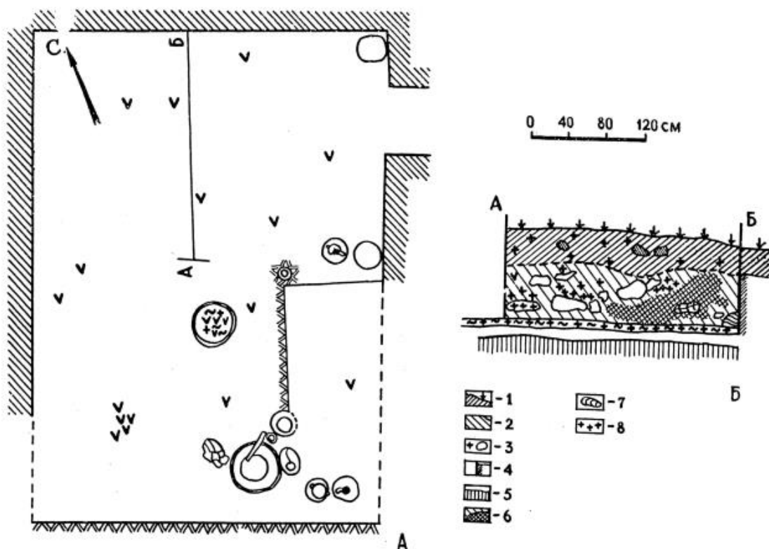
Расми 17. Ёдгории Чортеппа. Нақшаи ҳуҷраи № 1: А – нақша, Б – буриши археологӣ. (аск аз Е.П. Денисов, манба Археологические работы в Таджикистане Вып. 16. – С.96-105)
