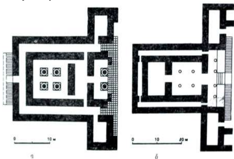
Расми 4. Лоиҳаҳои маъбади оташ:
