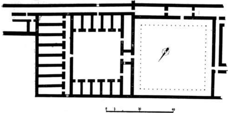
Расми 11. Ойхонум. Хазина. Лоиха
