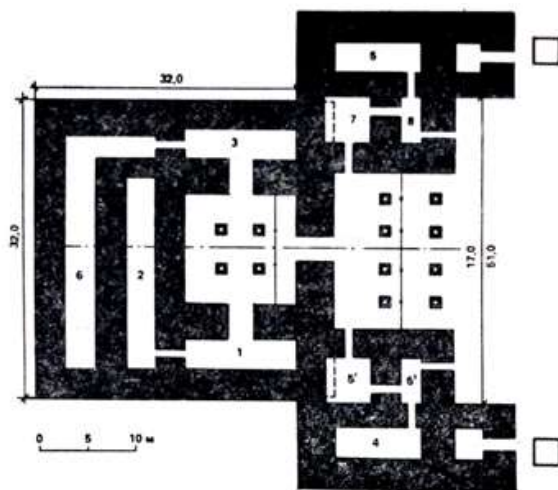
Расми 2. Нақшаи маъбади Омӯ. Асрҳои IV–III то милод
