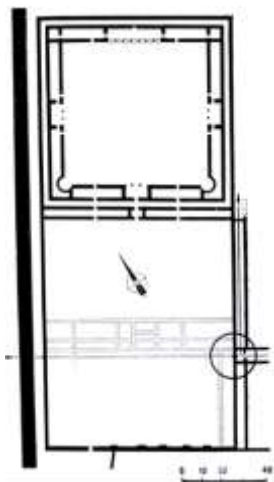
Расми 12. Ойхонум. Нақшаи омӯзишгоҳ.
