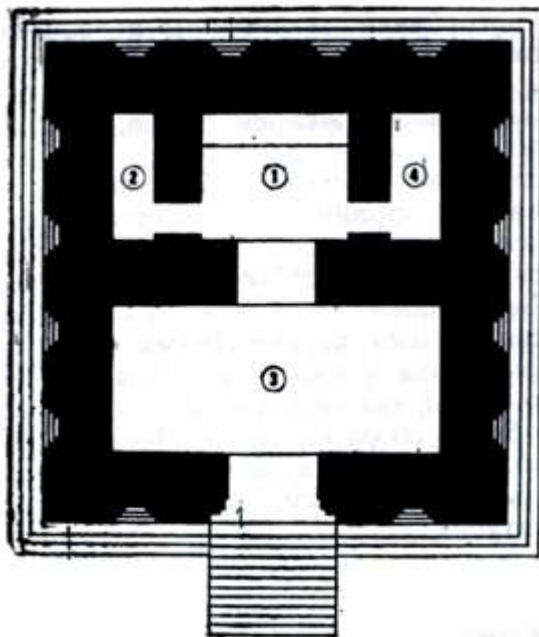
Расми 15. Ойхонум. Нақшаи маъбад бо тоқчаҳои зинадор.
